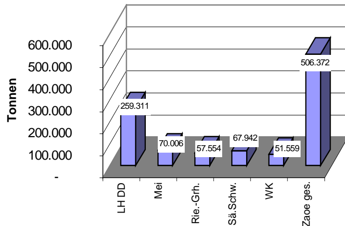
Abb. 1: Siedlungsabfallaufkommen 1999
